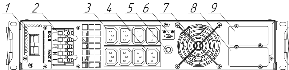
Рисунок 11. Компоненты задней панели ИБП Штиль STR1103TL
