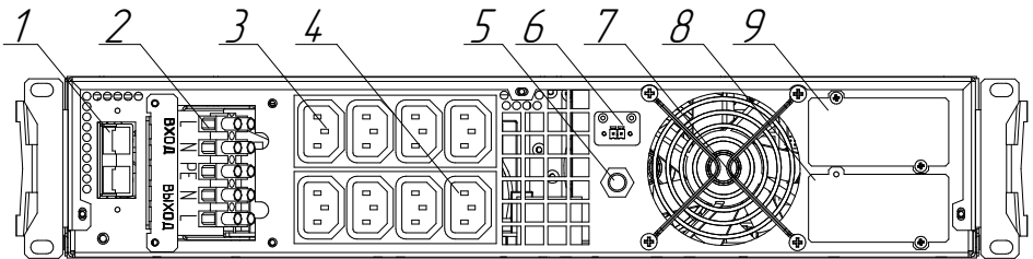
Рисунок 9. Компоненты задней панели ИБП Штиль STR1103TLD
