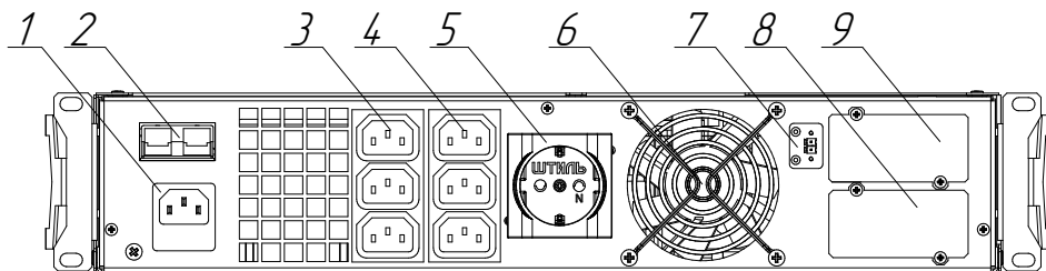
Рисунок 7. Компоненты задней панели ИБП Штиль STR1101L, STR1101SL и STR1101LD
