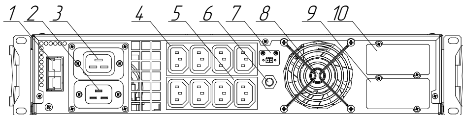
Рисунок 10. Компоненты задней панели ИБП Штиль STR1102L и STR1103L
