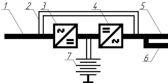
Рисунок 14. Компоненты мнемосхемы
