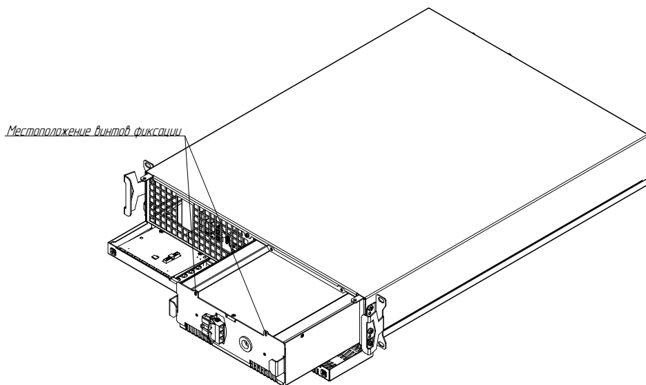
Рисунок Б3. Извлечение батарейного блока из ИБП Штиль STR1102SL и STR1103SL.
