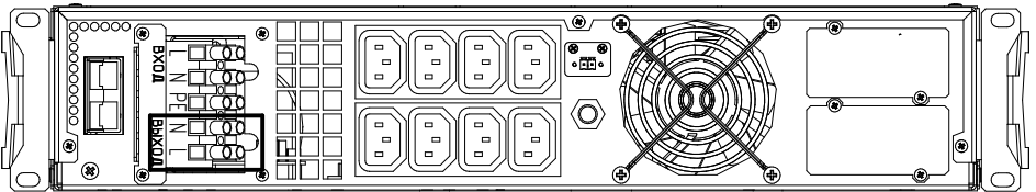
Рисунок 18б. ИБП Штиль STR1103TL. Выводы «Выход N-L»
