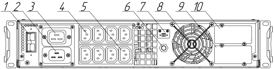
Рисунок 8. Компоненты задней панели ИБП Штиль STR1102SL, STR1102LD и STR1103SL
