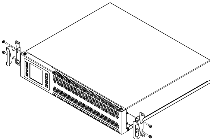
Рисунок 15. Установка кронштейнов для горизонтального крепления у ИБП Штиль STR1101L, STR1101SL и STR1101LD 4
