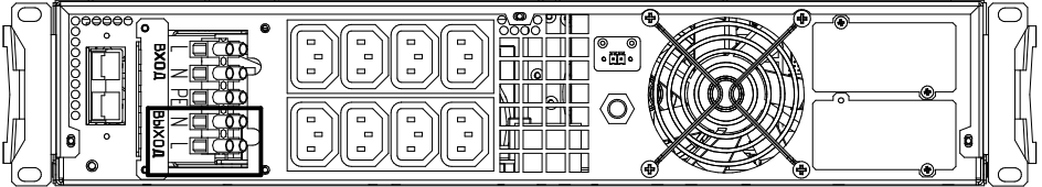
Рисунок 18а. ИБП Штиль STR1103TLD. Выводы «Выход N-L»
